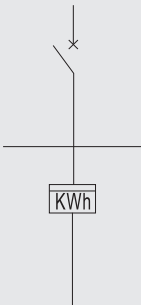
三相直通计量箱接线图
