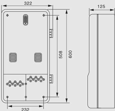
安装尺寸图(mm)
